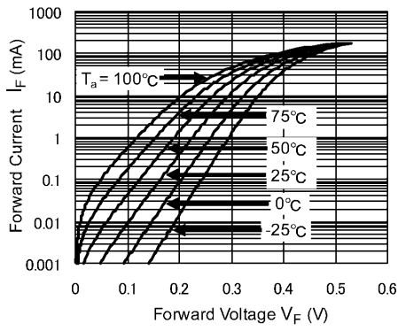
Fig. 9.1 I_F - V_F
