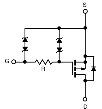
P-Channel MOSFET
