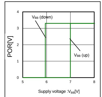
Figure 17. POR Threshold Voltage (Ta = 25 °C)
