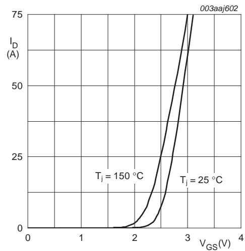
V_{DS} = 10V
