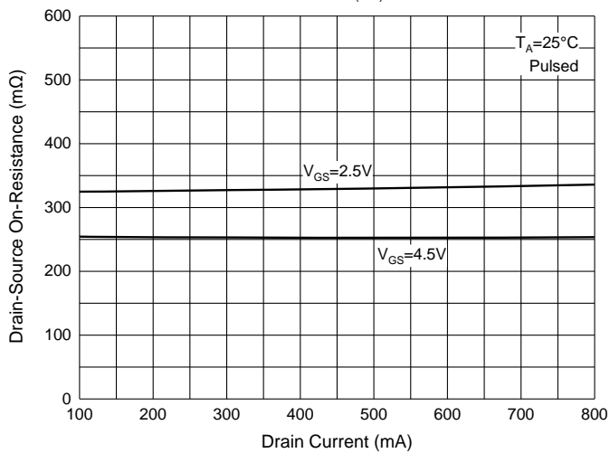
Fig. 3 - R_{DS(ON)} - I_D
