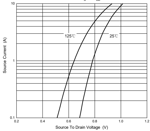
Fig. 9 - I_S - V_{SD}
