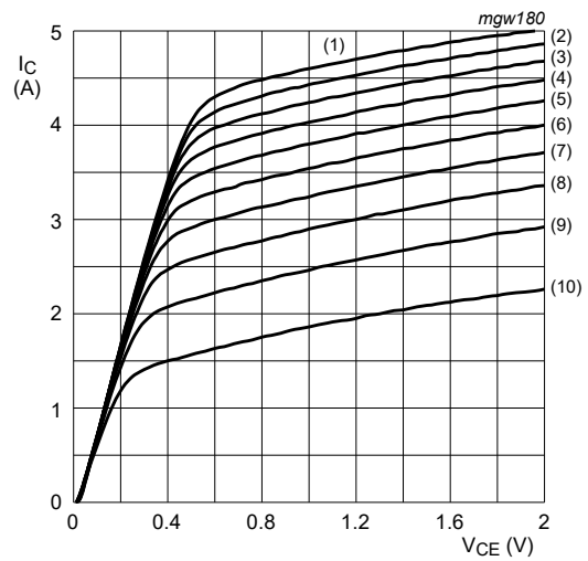
T_{amb} = 25\text{ }^\circ\text{C} (1) I_B = 150\text{ mA} (2) I_B = 135\text{ mA} (3) I_B = 120\text{ mA} (4) I_B = 105\text{ mA} (5) I_B = 90\text{ mA} (6) I_B = 75\text{ mA} (7) I_B = 60\text{ mA} (8) I_B = 45\text{ mA} (9) I_B = 30\text{ mA} (10) I_B = 15\text{ mA}
