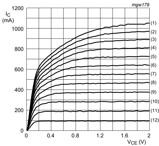
T_{amb} = 25\text{ }^\circ\text{C} (1) I_B = 3.96\text{ mA} (2) I_B = 3.63\text{ mA} (3) I_B = 3.30\text{ mA} (4) I_B = 2.97\text{ mA} (5) I_B = 2.64\text{ mA} (6) I_B = 2.31\text{ mA} (7) I_B = 1.98\text{ mA} (8) I_B = 1.65\text{ mA} (9) I_B = 1.32\text{ mA} (10) I_B = 0.99\text{ mA} (11) I_B = 0.66\text{ mA} (12) I_B = 0.33\text{ mA}
