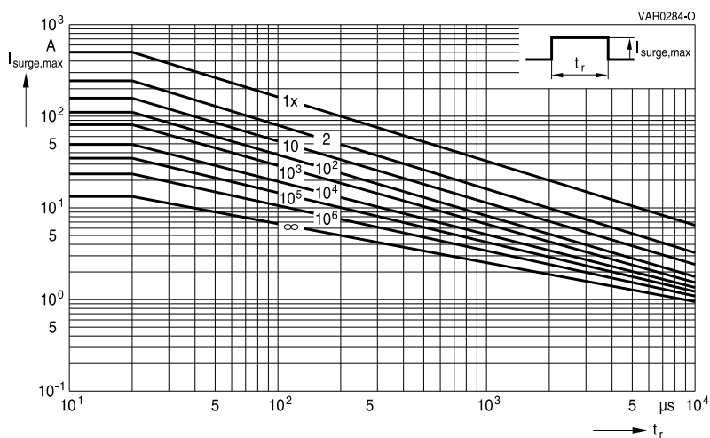
CN1812M4G ... M6G
