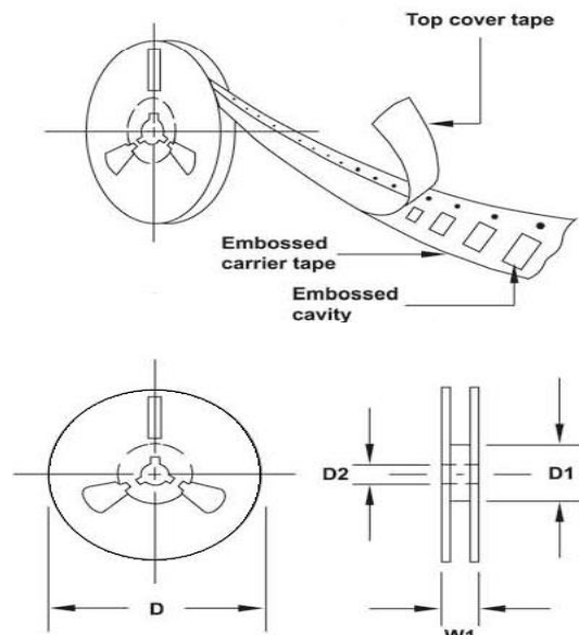
DO-214AC(SMA) - Reel
