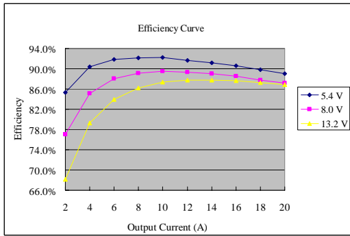
Vo=1.5 V
