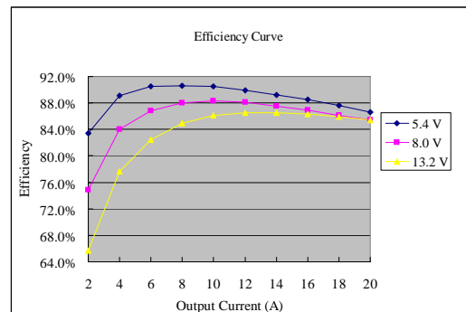
Vo=1.2 V
