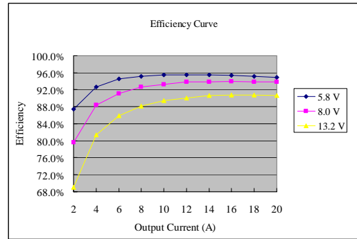
Vo=3.3 V
