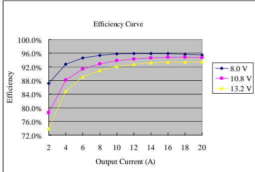
Vo=5.5 V
