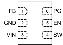
UDFN-6L 1.4x1 (FC)
