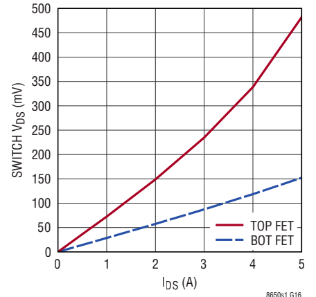
Switch V_{DS}
