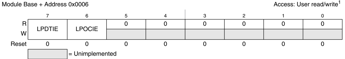
Figure 15-9. LIN Interrupt Enable Register (LPIE)
