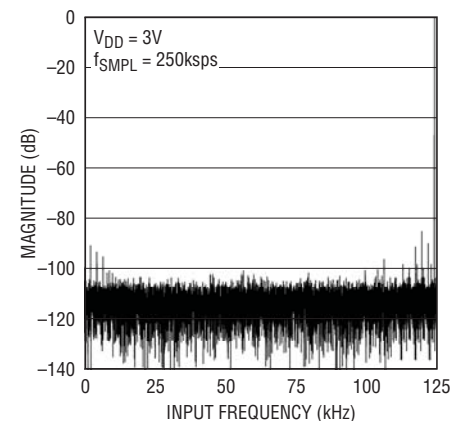
124kHz Sine Wave 8192 FFT Plot
