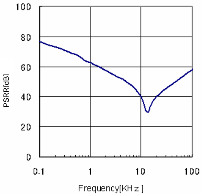
Fig.20 PSRR ( I_o=0 mA)
