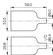
PNo 11987
