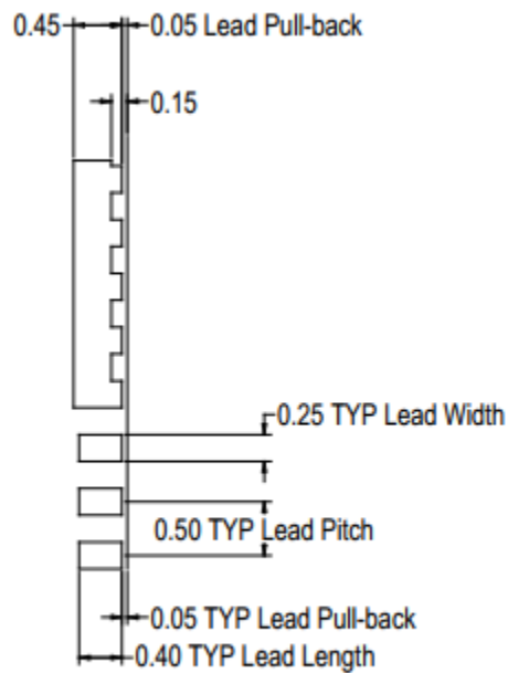
DETAIL A SCALE: 2x
