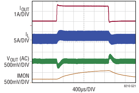
Load Step (Buck Region – Figure 37)
