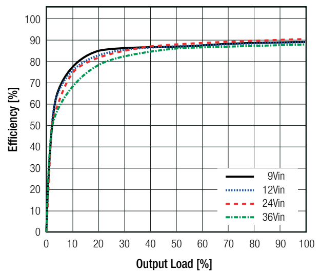
REC15E-2412SZ
