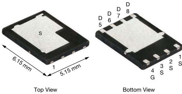
PowerPAK® SO-8DC
