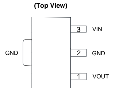
SOT89
