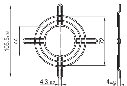
LZ22-N Fan size 80 x 80
