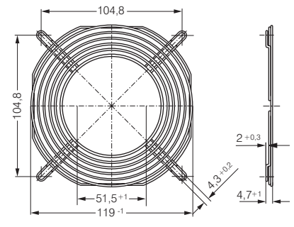
LZ30-9 Fan size 119 X 119
