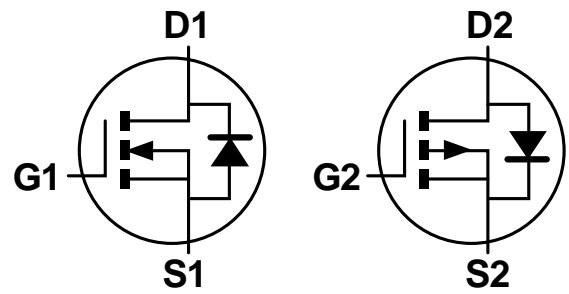
Q1 N-Channel
