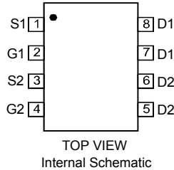
SO-8
