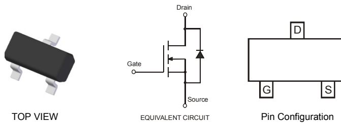
SOT-23
