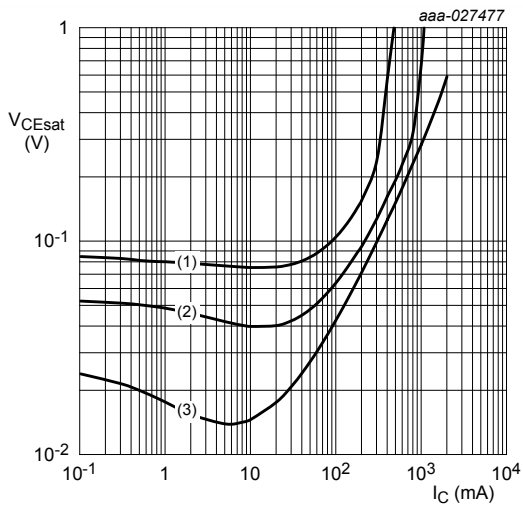
T_{amb} = 25^\circ\text{C} (1) I_C/I_B = 50 (2) I_C/I_B = 20 (3) I_C/I_B = 5
