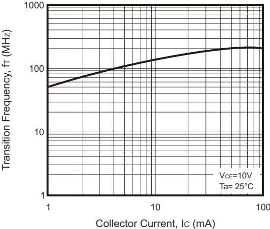
Fig.7 - f_T — I_C
