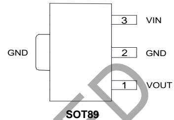
SOT89
