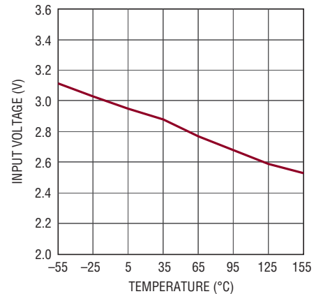
V_{IN} UVLO
