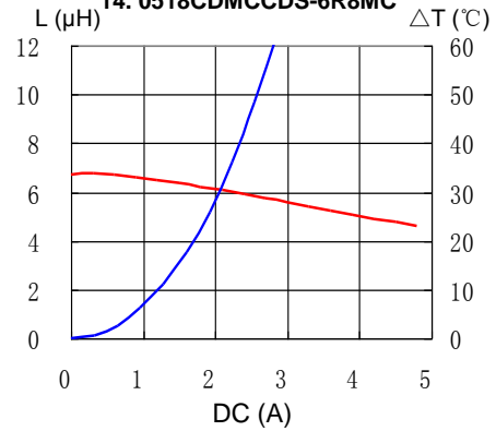
14. 0518CDMCCDS-6R8MC
