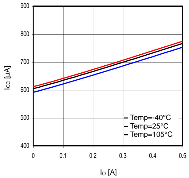
Fig. 30 I_o - I_{cc}
