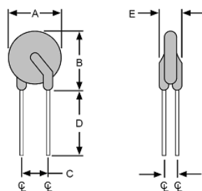
FRX 110-90F ~ FRX 375-90F
