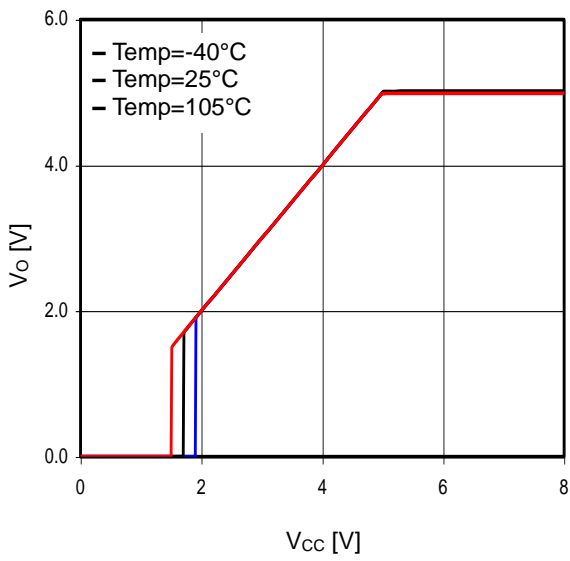
Fig. 27 V_{cc} - V_o ( I_o=0\text{mA} )
