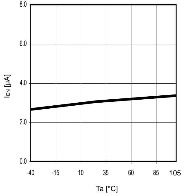
Fig. 24 Ta- I_{EN}
