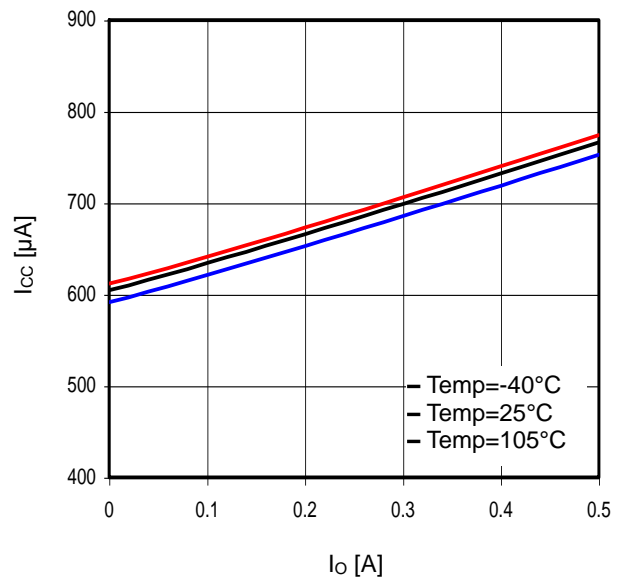
Fig. 30 I_o - I_{cc}
