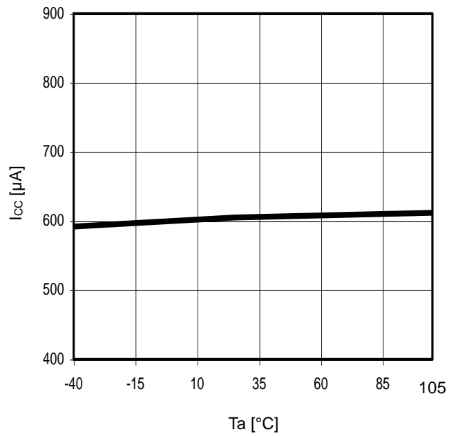
Fig. 22 T_a - I_{CC}
