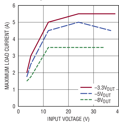
Maximum Load Current vs VIN \text{BIAS} Open
