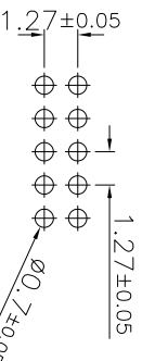
P.C.B Layout
