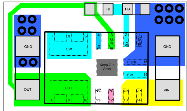
Top Layer
