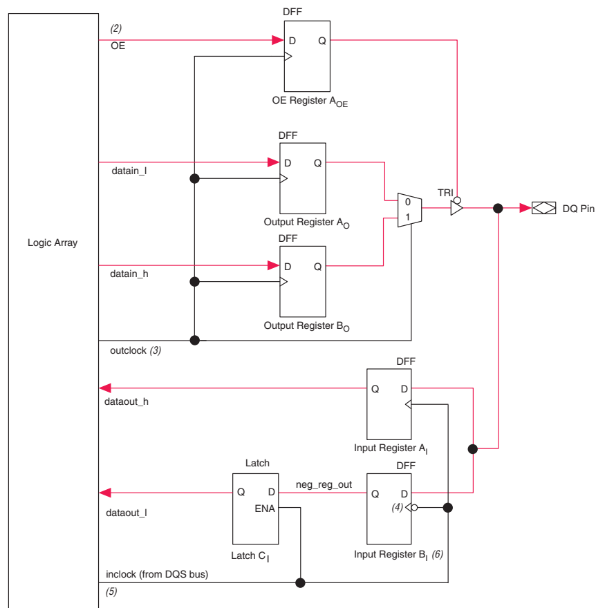
Figure 3–15. DQ Configuration in Stratix II or Stratix II GX IOE Note (1)
