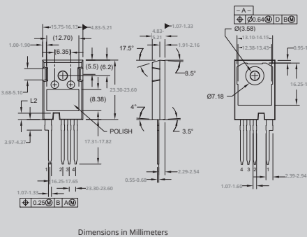
TO-247-4L Notch
