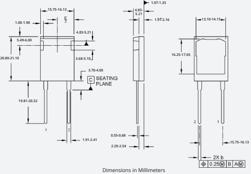
T-MAX®
