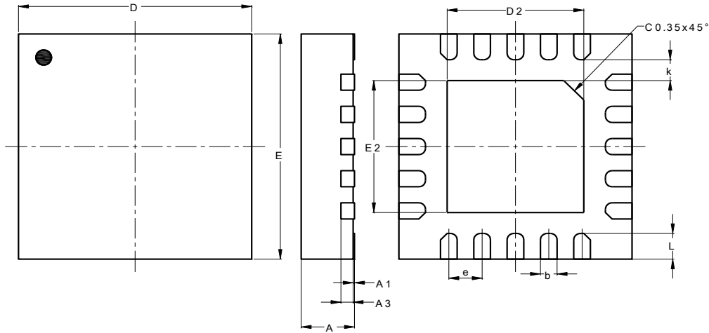
W-QFN3535-20 (Type A1)
