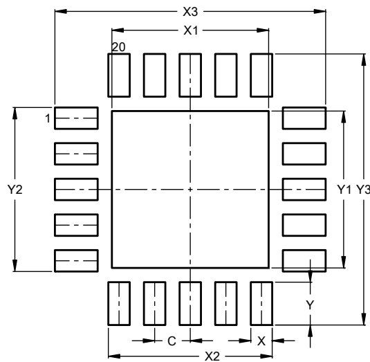
W-QFN3535-20 (Type A1)
