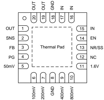
W-QFN3535-20 (Type A1)
