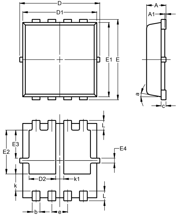
PowerDI3333-8 (Type UXC)
