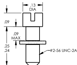
#2/56 M83513/05-03
