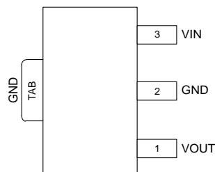
SOT89
