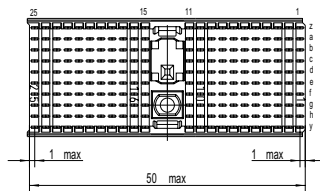
Lochbild fuer Leiterplatte (Bestückungssseite)
