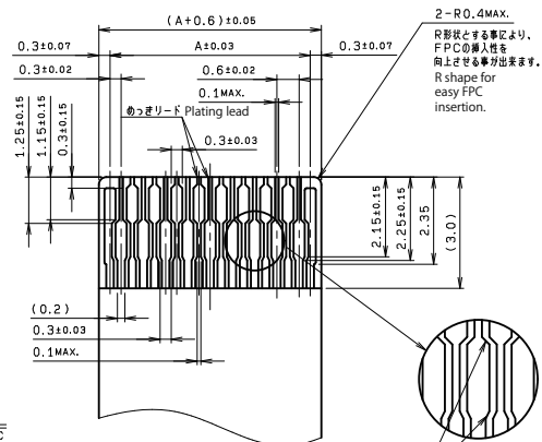
支持テープ SUPPORTING TAPE 適用FPC寸法 APPLICABLE FPC
