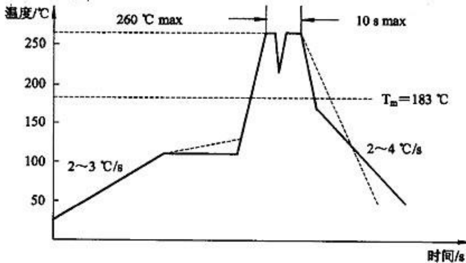
双波峰焊的典型温度曲线
