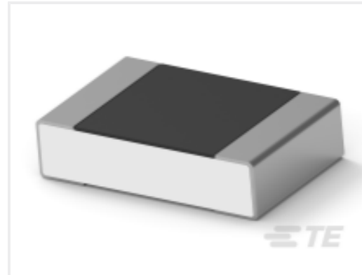
TE Part #5-2176375-5 RQ 0805 4K22 0.1% 10PPM 1K RL
