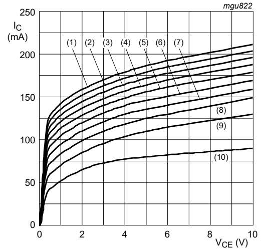
T_{amb} = 25\text{ °C} (1) I_B = 5.0\text{ mA} (2) I_B = 4.5\text{ mA} (3) I_B = 4.0\text{ mA} (4) I_B = 3.5\text{ mA} (5) I_B = 3.0\text{ mA} (6) I_B = 2.5\text{ mA} (7) I_B = 2.0\text{ mA} (8) I_B = 1.5\text{ mA} (9) I_B = 1.0\text{ mA} (10) I_B = 0.5\text{ mA}
