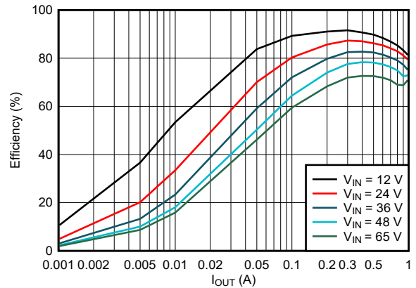
f_{SW} = 1.1\text{ MHz} V_{OUT} = 5\text{ V} LMR51610YF
