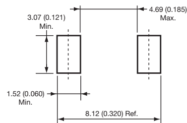
DO-214AB (SMC)
