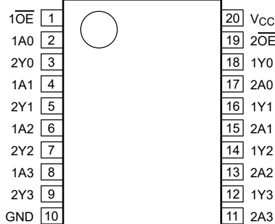
PW package SOT360-1 (TSSOP20)
